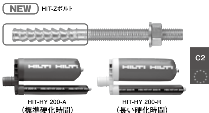
C2認証試験では地震加力の模擬状況かつひび割れのある状態で最大耐力と変位を確認します
