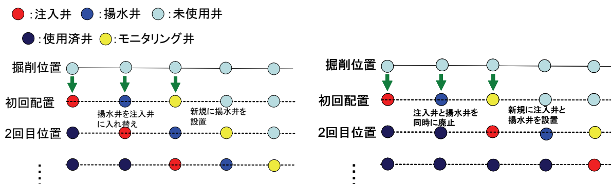
図 2.2.2-4 直線的な井の配置例
