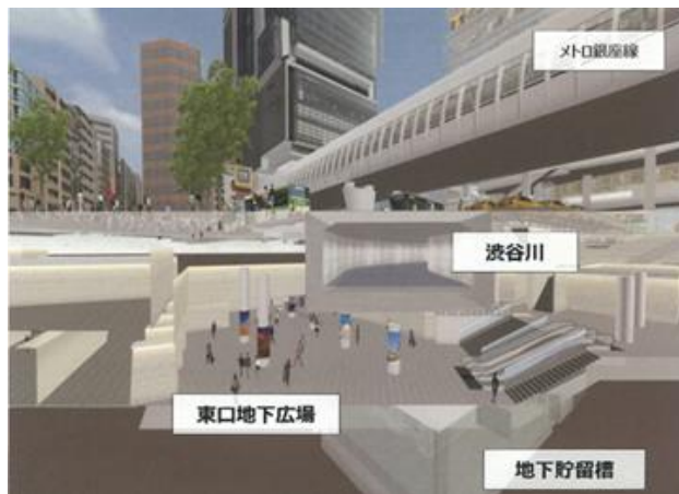
渋谷駅東口立体整備イメージ
