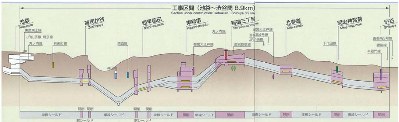
東京メトロ副都心線（13号線）工事区間の平面図および縦断面図 (出典；東京メトロ副都心線 パンフレット)
