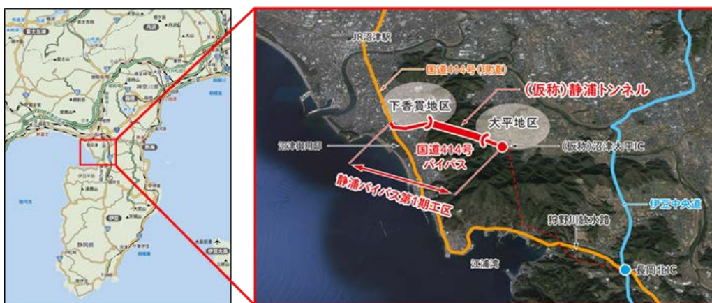
工事場所位置図 (工事概要資料より引用)
