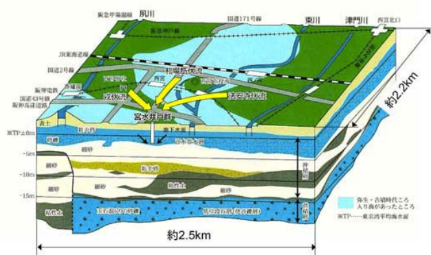
図 2.1.2-7 西宮市南部帯水層模式図（宮水地帯付近） （スミカワ研究所提供：無断転載厳禁）
