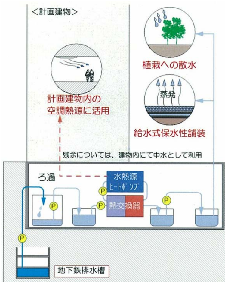
図 2.1.5-3 地下鉄湧出水活用イメージ図
