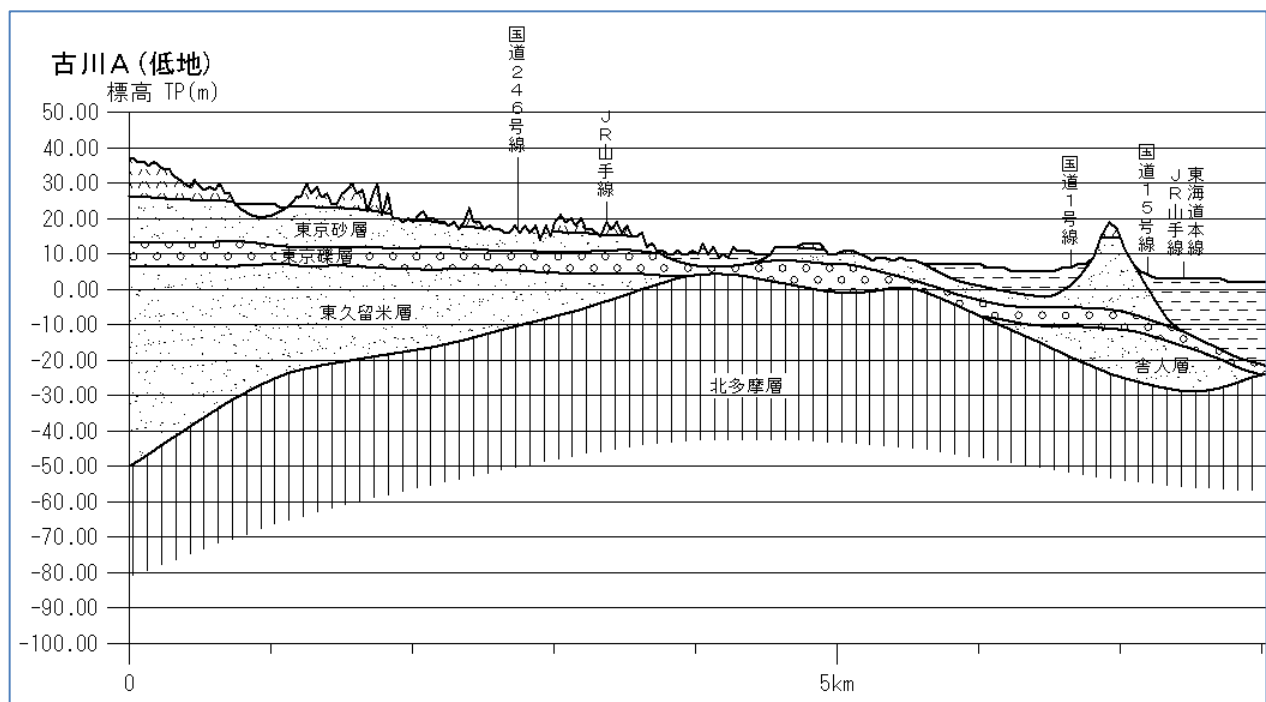
図 3.4.2-4(2) 六本木-溜池区域周辺の地質断面 東京都土木技術研究所(1996)東京都(区部)大深度地下地盤図を基に 作成
