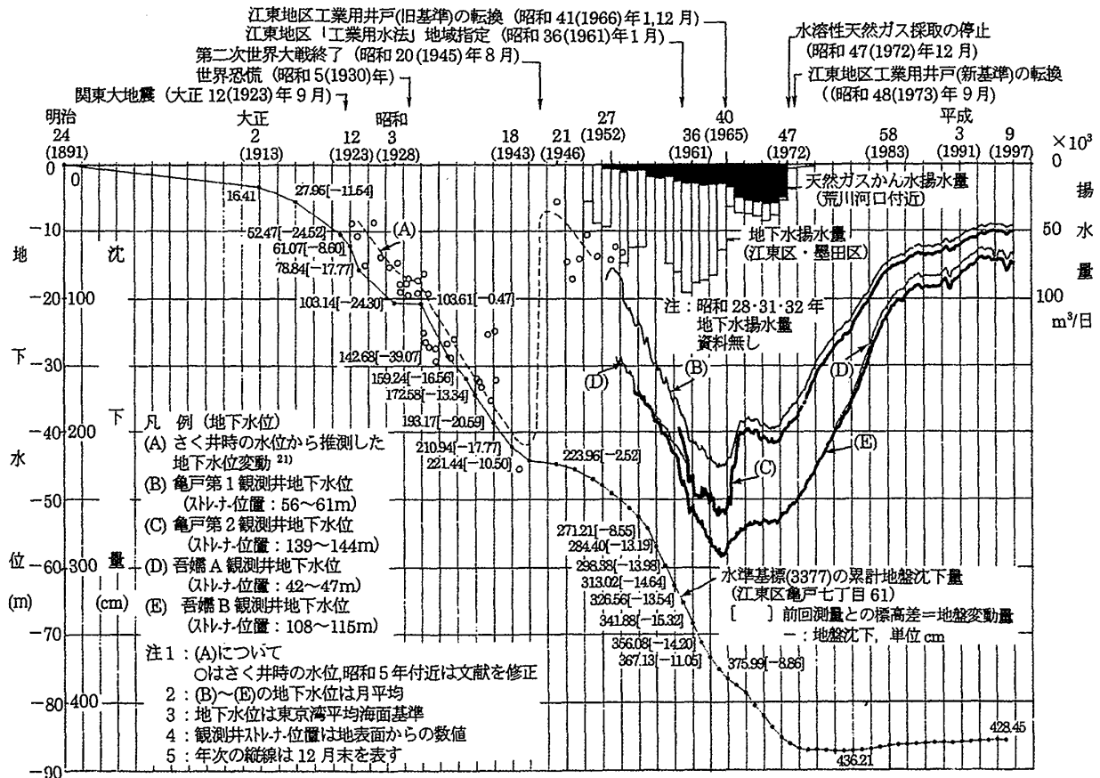
図 2.2.2-6 東京地域における地下水・天然ガスかん水の揚水量と被圧滞水層に設置した観測井の井戸内水位、地盤沈下量の推移
