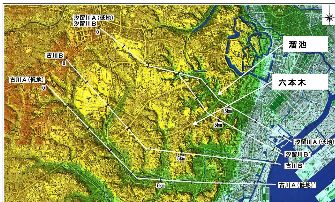
図 3.4.2-2 水文地質断面の検討位置
