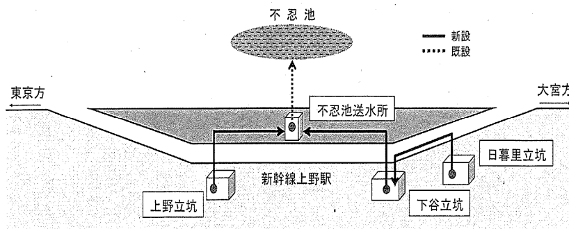
図 2.3-4-1 JR 上野地下駅周辺～不忍池への導水状況(清水満、2004 より引用)
