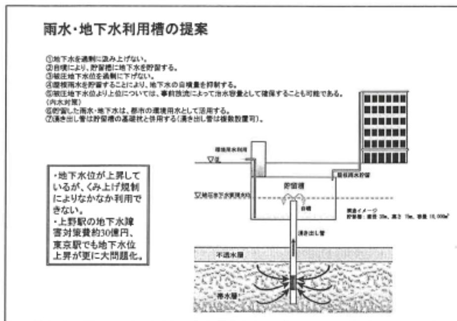
図-3.5.1-1 雨水・地下水利用槽の提案（雨水貯留浸透技術協会）
