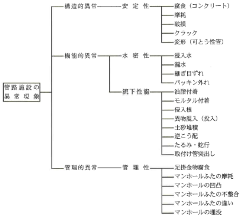
図 3.8.2-1 管路施設の異常現象の例
