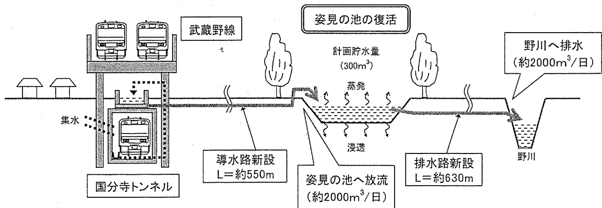
図 2.3.5-1 JR 武蔵野線国分寺トンネルにおける湧水活用事例（清水，2004 より引用）
