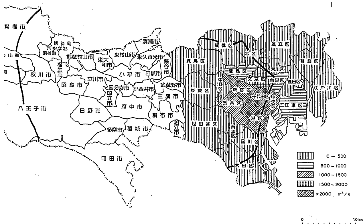
図 2.2.2-7 区別の地下鉄・洞道への地下水湧出量
