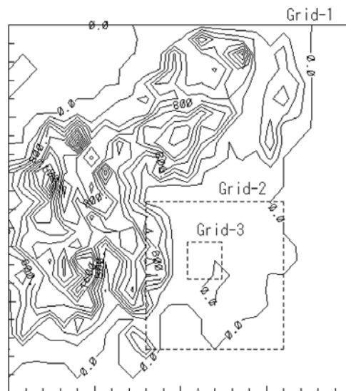
図 2.4.3-1 解析に用いた格子システム。Grid-3 には建物キャノピーの影響を考慮。
