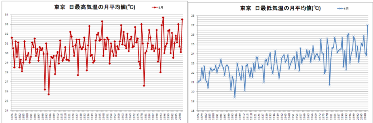
図 2.2.2-1 東京の日最高・低気温の 8 月平均値の推移
