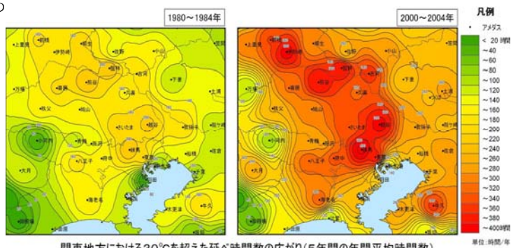
図 3.3.1-1 関東地方における 30℃を超えた延べ時間数の広がり (5年間の年間平均時間数) 出典：環境省 HP
