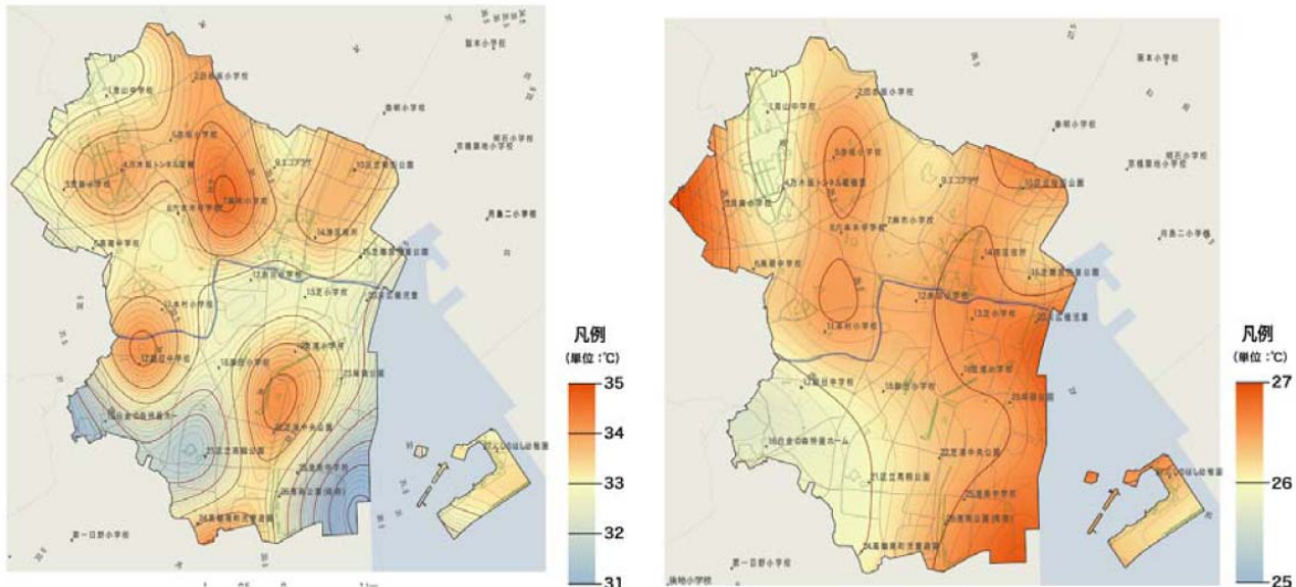
図 2.2.2-3 2007 年 8 月の日最高及び最低気温平均値図
