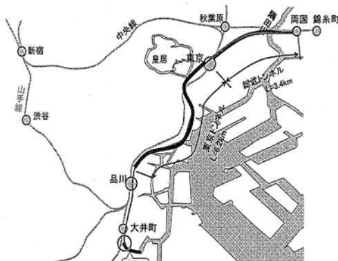
図 2.3.4-2 JR 総武線東京駅周辺～立会川への導水状況(清水満、2004 より引用)
