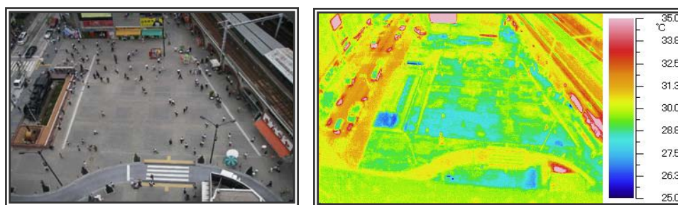
図 2.4.1-3 保水性舗装による表面温度上昇抑制効果(新橋 SL 広場)(出典:港区提供資料)
