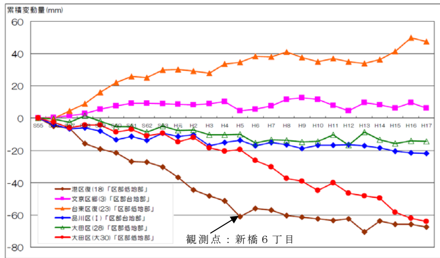
図2.2.2-11 水準基標 6 地点における累積地盤変動量
