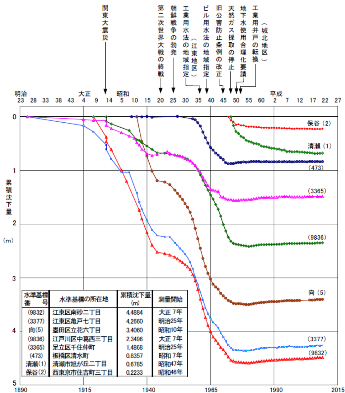
図 2.2.2-10 主要水準基標の累積沈下量図
