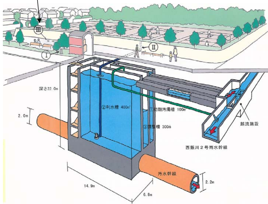
図 2.1.3-2 施設概要図
