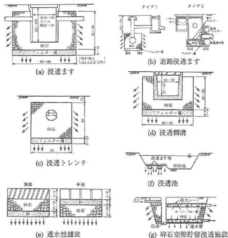
図 2.4.1-5 雨水浸透施設の手法例（東京都，2002）
