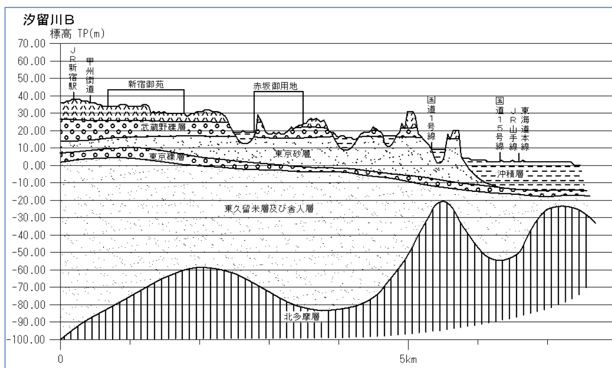
図 3.4.2-4(1) 六本木-溜池区域周辺の地質断面 東京都土木技術研究所(1996)東京都(区部)大深度地下地盤図を基に 作成
