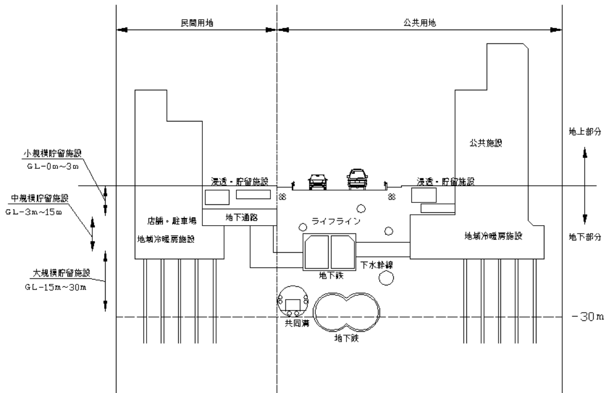
図 4.2.1-1 検討モデル一般図
