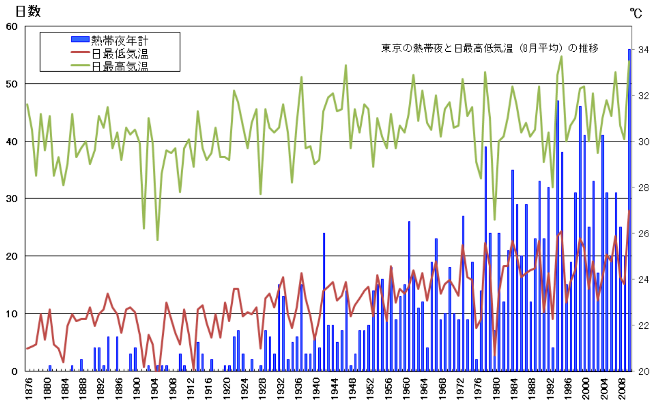
図 2.2.2-2 東京の熱帯夜と日最高低気温（8 月平均）の推移
