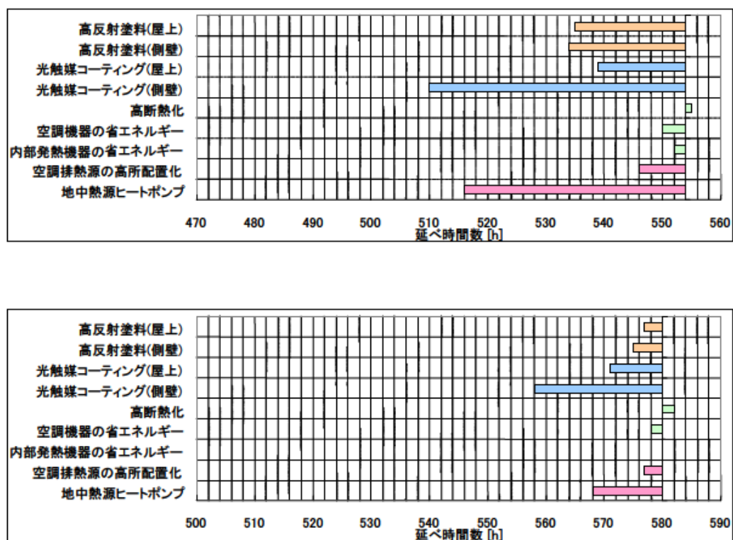
図 2.4.3-2 ヒートアイランド緩和対策技術による、夏季の日中における 30℃以上の気温が出現する延べ時間の低減効果（上）、および、夏季の夜間における 25℃以上の気温が出現する延べ時間の低減効果（下）
