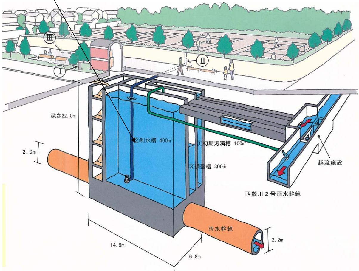
図 2.1.3-1 施設概要図
