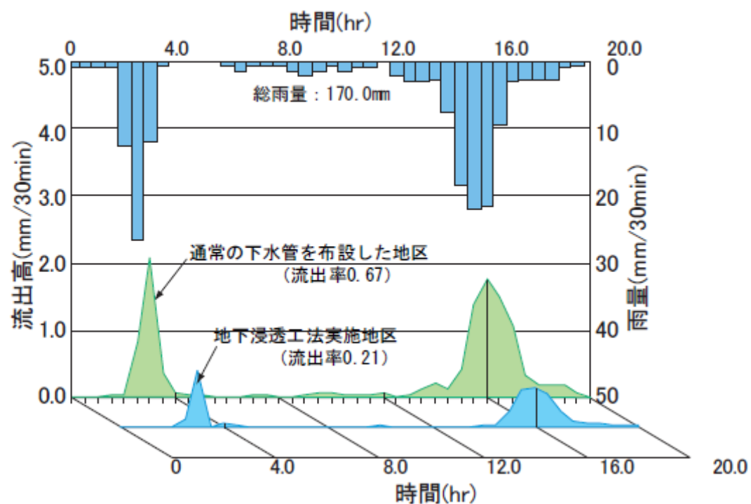
図 2.3.3-1 浸透施設による流出抑制効果 (雨水浸透貯留技術協会, 2007 より引用)
